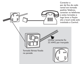
Figura 2 – Conexões Central PABX INNOVARE 2x8
